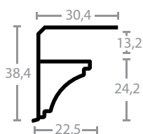
D ZÓCALO SANITARIO J
